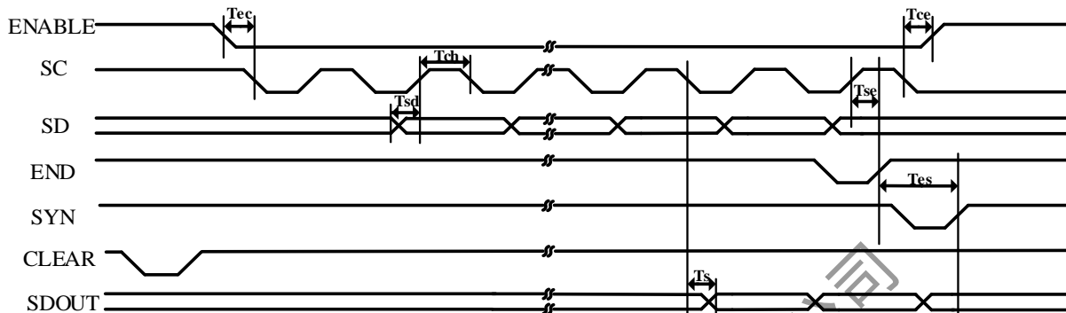
图 8 串行接口时延图
