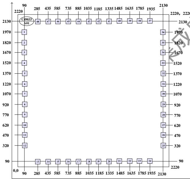
图 2 C49033 引脚分布图
