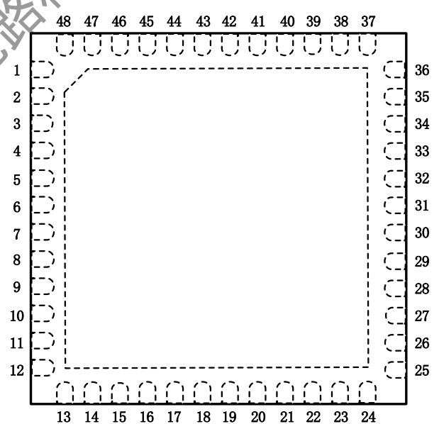
图 3 C49033T 引脚分布图
