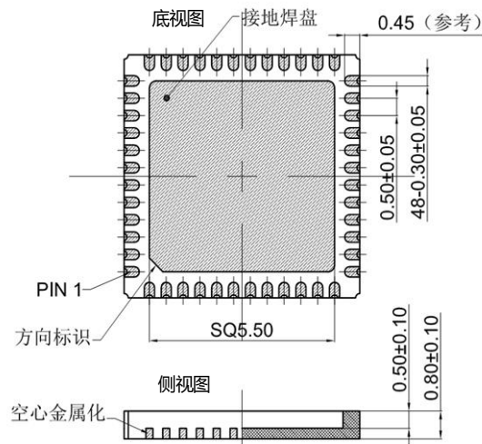
图 10 C49033T 底视图、侧视图
