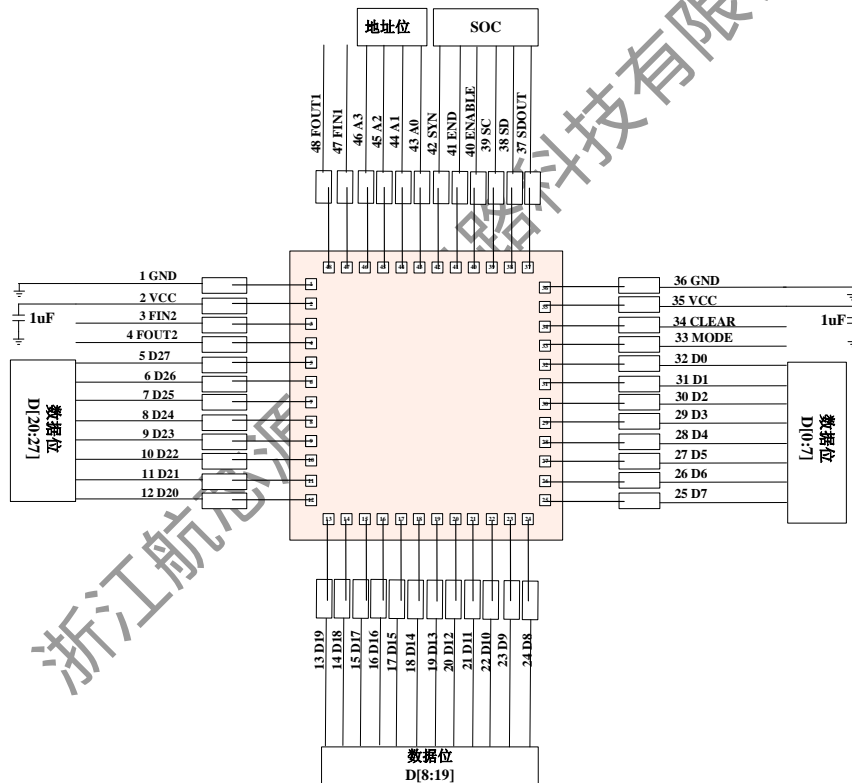
图 9 C49033 工作推荐电路
