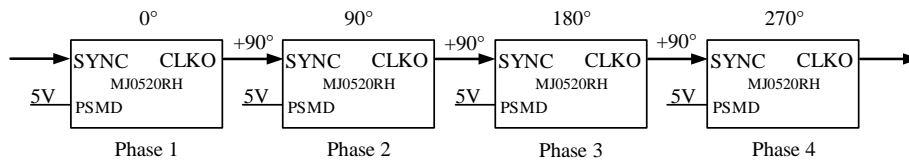
图 13 4 路并联连接示意图
