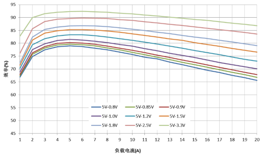
图 9 MJ0520RH 效率转化曲线
