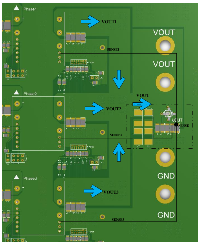
图 16 并联应用 pcb layout 示意图 1
