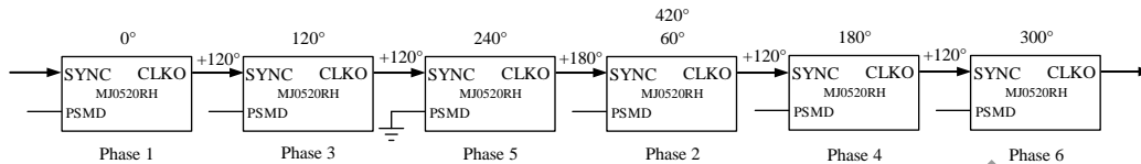
图 14 6 路并联连接示意图
