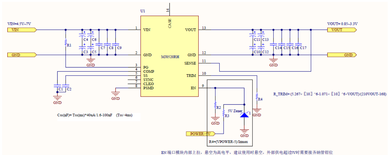
图 10 模块单路典型应用图
