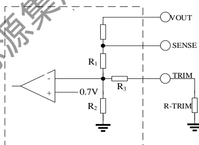
图 3 反馈网络示意图
