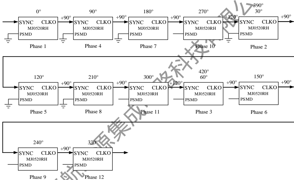
图 15 12 路并联连接示意图
