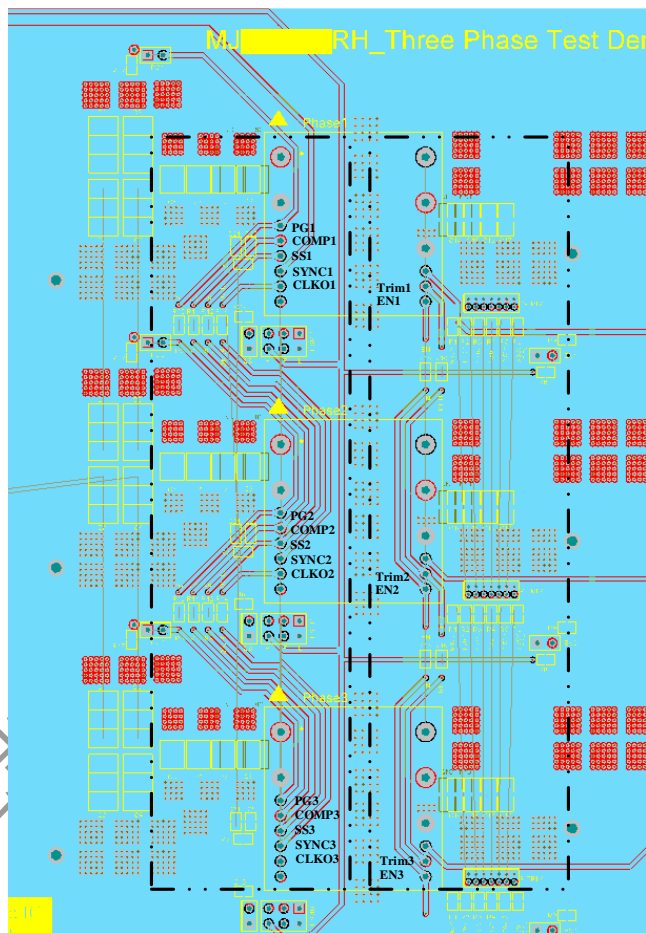
图 17 并联应用 pcb layout 示意图 2
