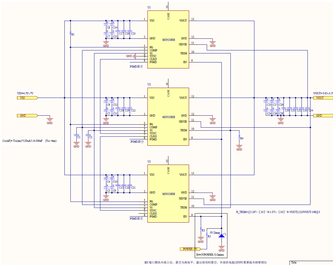
图 12 三路并联应用原理图
