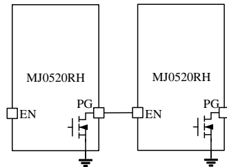
图 5 顺序启动
