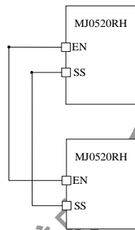
图 6 同时启动
