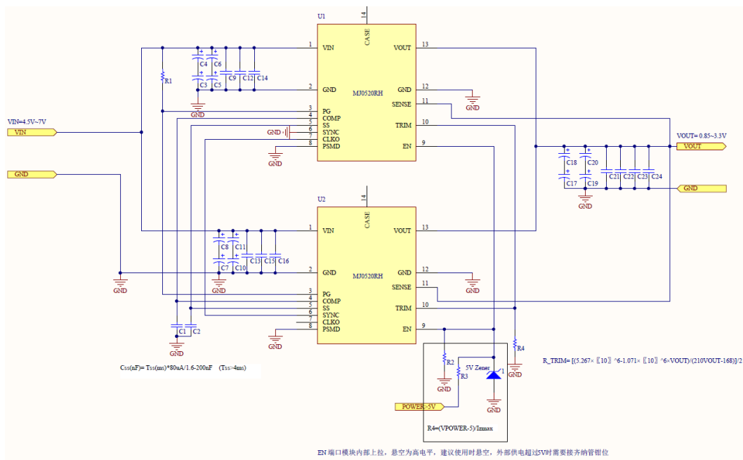
图 11 MJ0520RH 双路并联推荐应用电路
