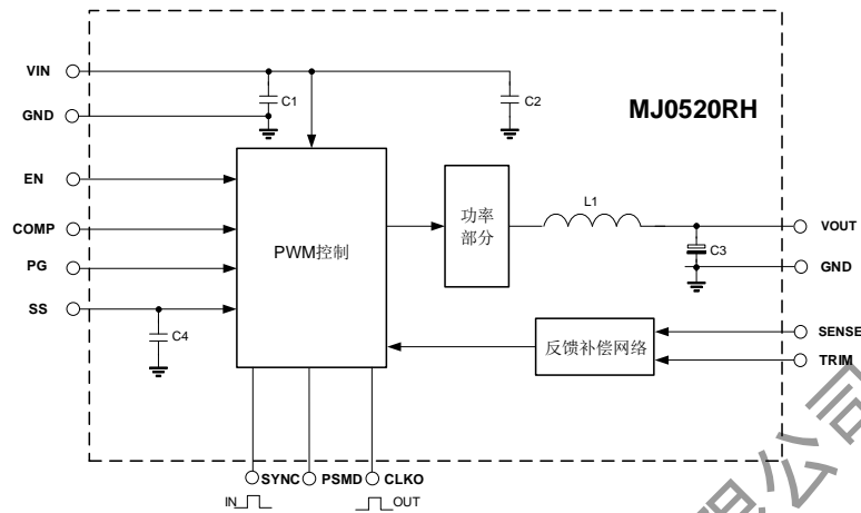
图 1 MJ0520RH 模块框图
