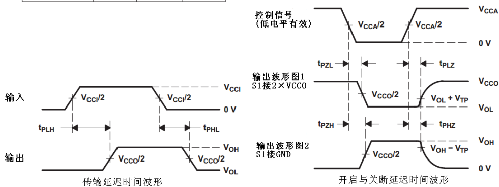
图 1 负载电路和波形图
