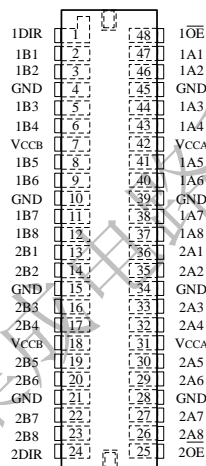
图 2 C45003RHO 脚位图(顶视图)
